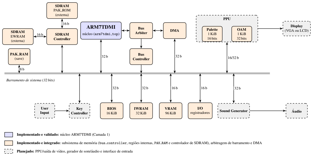
Figura 7: Arquitetura-objetivo do projeto. O núcleo ARM7TDMI (azul) já se encontra implementado e validado; o subsistema de memória (laranja), bus_controller, regiões internas (BIOS, IWRAM, VRAM, I/O, Palette, OAM), PAK_RAM e o controlador da SDRAM externa, que abriga a PAK_ROM e a EWRAM, além da arbitragem de barramento e dos quatro canais de DMA, encontra-se implementado e integrado ao datapath , com a validação funcional do caminho integrado ainda em andamento; os blocos de PPU e saída de vídeo, gerador de som e áudio, e a interface de entrada ( Key Controller ) permanecem planejados (cinza). As larguras indicadas correspondem ao barramento nominal de cada região; a decodificação por região emprega o nibble alto do endereço ( addr[27:24] ).
